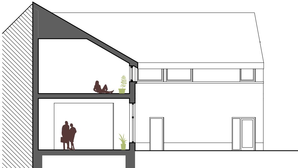
B-B
